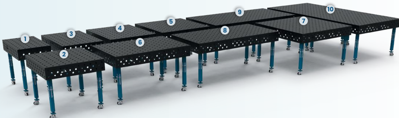
DIMENZIJE EXPERT, PRO, PLUS I ECO STOLOVA [mm].
